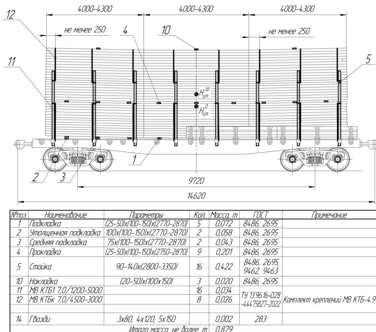
Рисунок 22 - Размещение и крепление непакетированного пиломатериала длиной 4,0-4,3 м на универсальной платформе с разделением штабеля на две части
