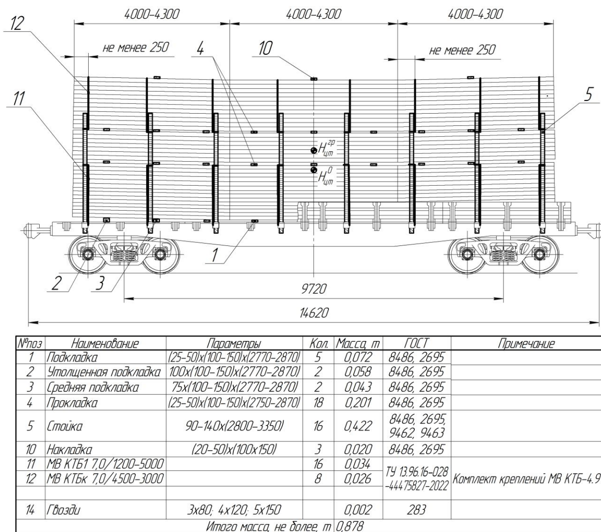
Рисунок 16 - Размещение и крепление непакетированного пиломатериала длиной 4,0-4,3 м на универсальной платформе с разделением штабеля на три части
