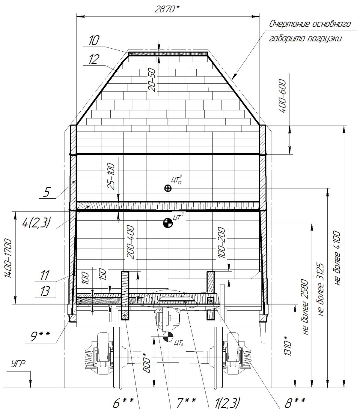
Рисунок 12 - Поперечное сечение непакетированного пиломатериала на платформе с разделением штабеля на две части прокладками.
